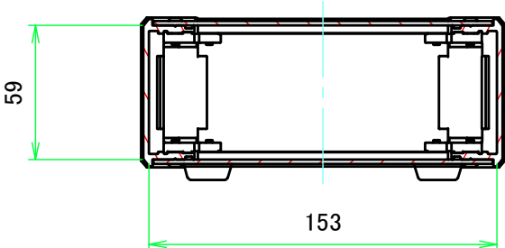
B-B ( 1:3 )
